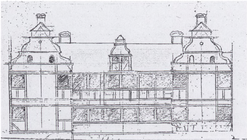
Fig. 4. Sydfacaden af Hans den Yngres slot. Rekonstruktion som foregående (jvf. fig. 10), her med overklistering af gavlpartiets stueetage i den vestre sidefløj.
