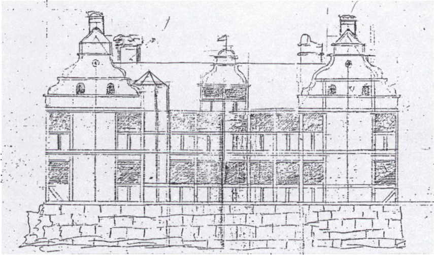
Fig. 3. Hans den Yngres slot. Facaden mod nord. Rekonstruktion på grundlag af bygningstegningen fra 1665 ved fraklipning af midterbygningens 3. stokværk samt påklistering af gavlkvisten og den øverste del af indgangstårnet (jfr. fig. 9).
