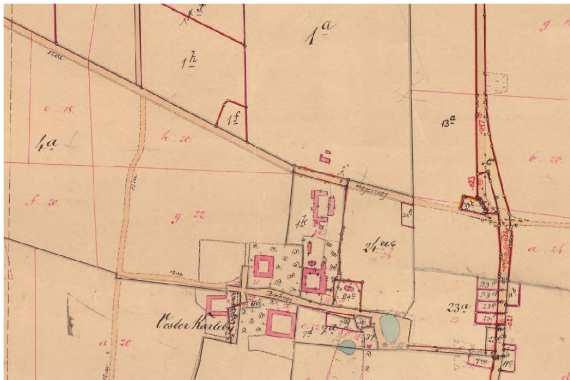
Matrikelkort 1882. Geodastystyrelsen.
