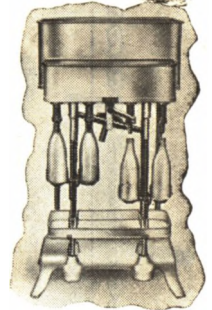
Tappemaskine med Beholder.
