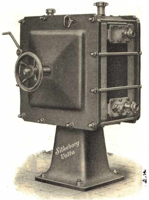
VOLTA Pladeapparat Model 1934.
