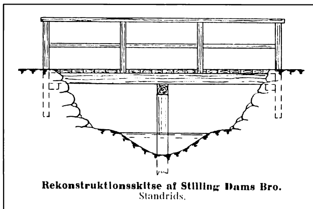
"Stilling Dams Bro". Snittegning af broen, som førte en bæk under Skanderborg Landevej i Kongsvang.
