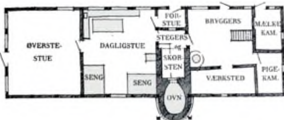
Grundplan over et sjællandsk husmandshus. Køkkenskorsten er i midten, hvorfra der fyres til alle ildsteder.
