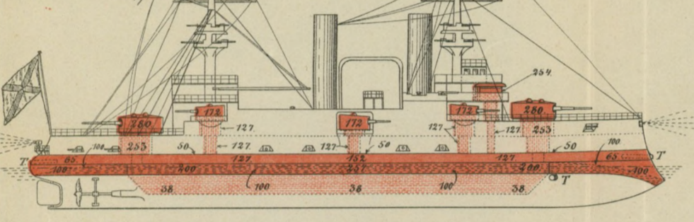
2 Stk. 3gangs Exp. Mask. 20 Kædler, Belleville Kullbeholdn. 1250 Tons. Aktionsrad m. 10 Knob - 5500 Kml.
