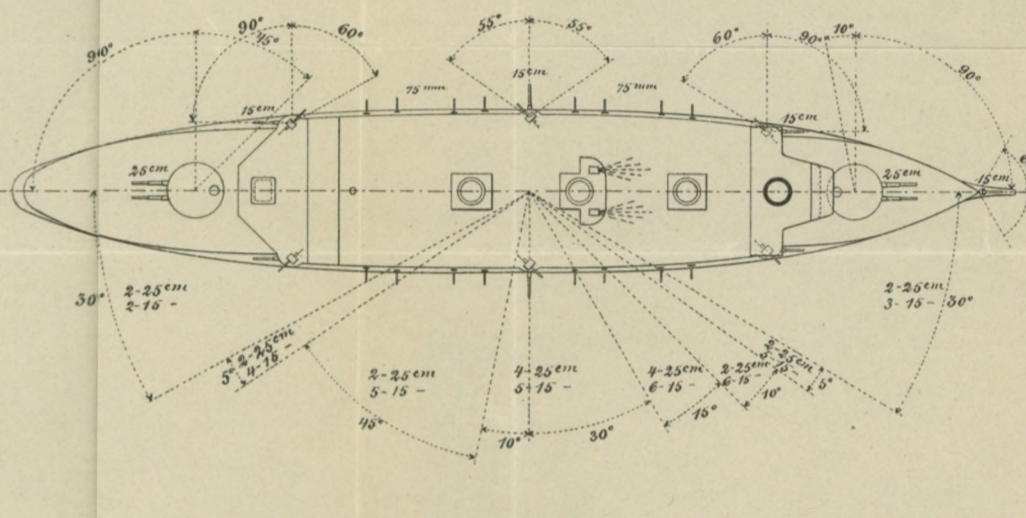
Samme Type Peresvet.....1898 Ostrobia.....1898 Vanselin - Russeret strækker sig kun over 1/3 af Skibets Længde.
