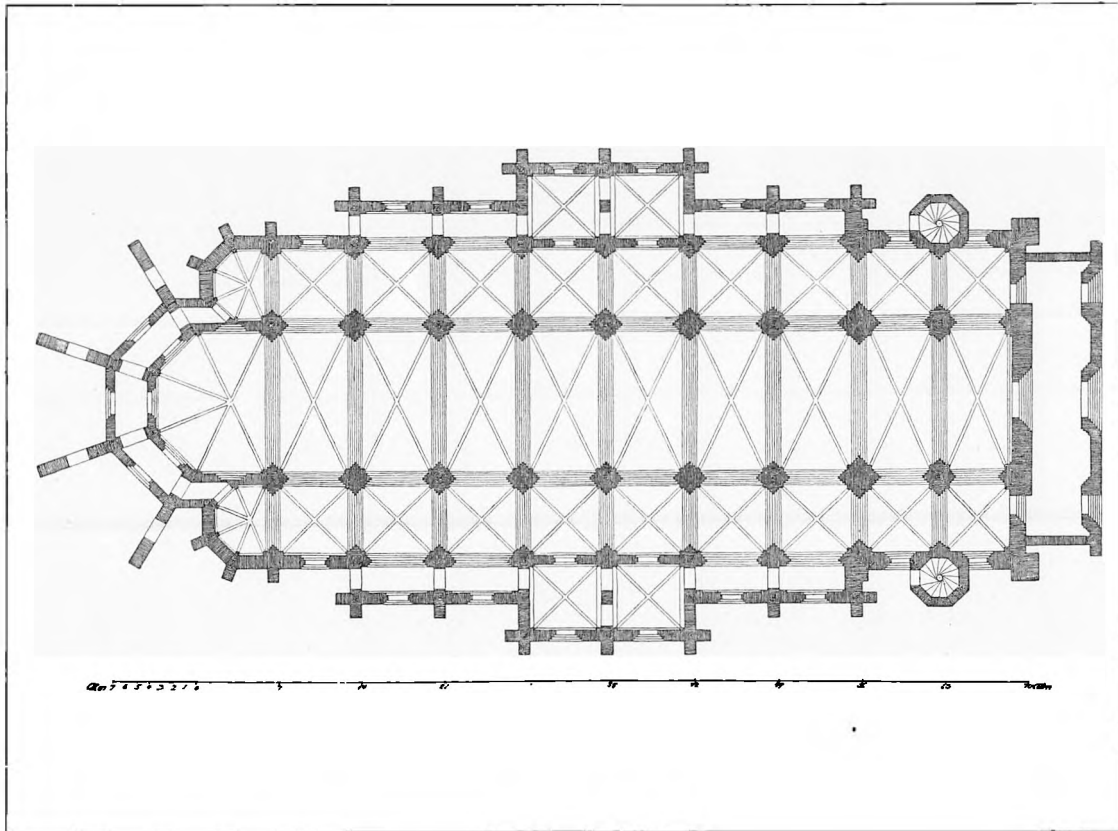
P. V. Jensen-Klint: Plan af Grundtvigs Kirken. 1913.
