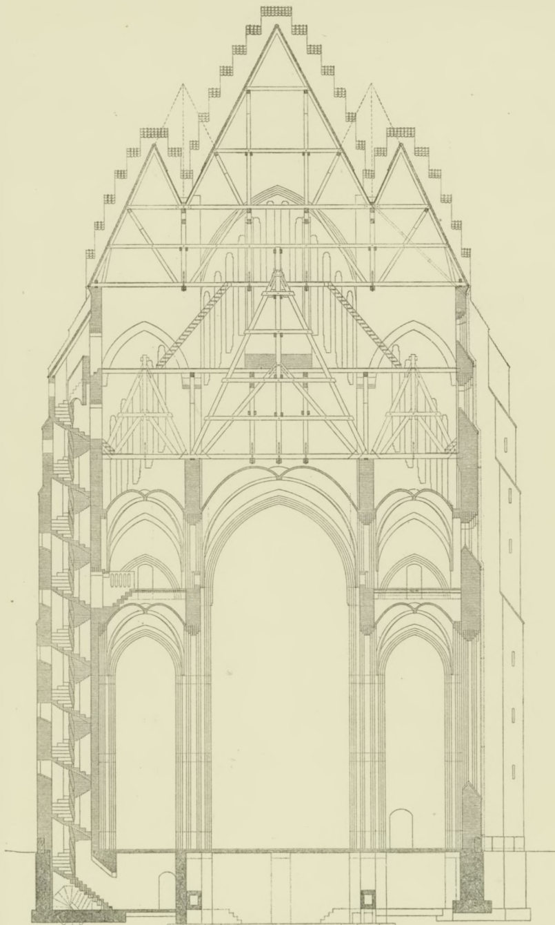
Rev. 3 o Feb. 1898 GRUNDTVIGS KIRKE CAARN: SNIT NORD-SYD. P. W. Jørgen Albert
