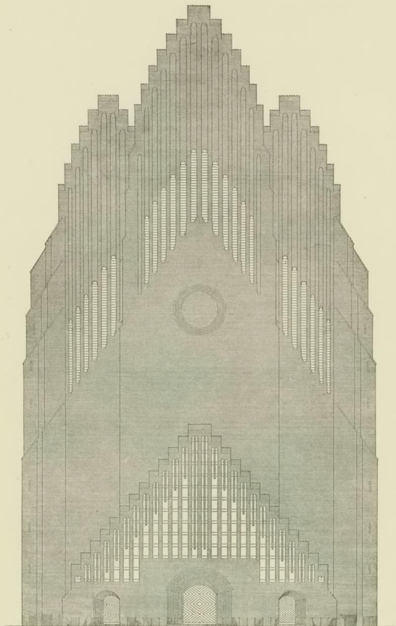
Rev. 16 o Sept. 1898 GRUNDTVIGS KIRKE CAARN: VESTSPRONCEN. P. W. Jørgen Albert
