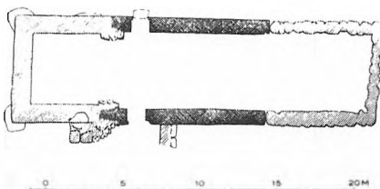
Vredsløse. Plan. 1:300. Maalt af K.V. Barfoed 1916.
