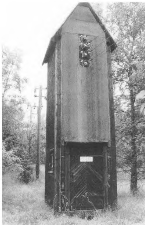
Transformerstation nr. 201. Elmuseet, Tange.
