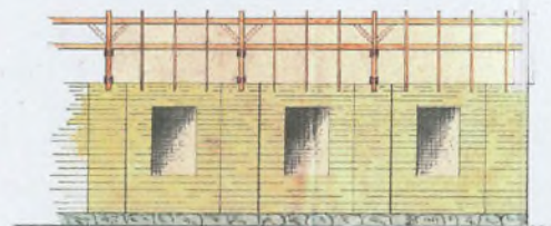
Lage der Sparren. 1:100
