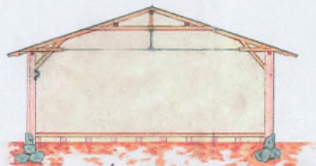
Schnitt A B
