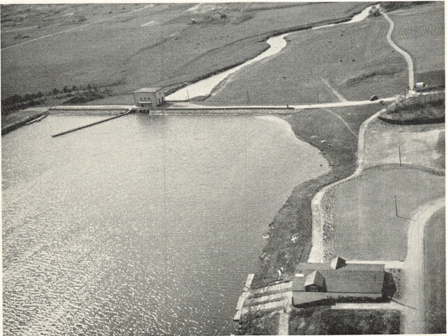
Under besættelsen blev Storaen lagt i arbejdselen. Det store vandkraftanlæg krævede en vældig opdæmning, og en stor sø blev skabt. I forgrunden ses kajakroernes klubhus.
