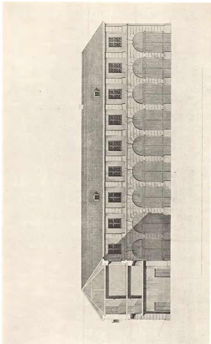
Fig. 5. Den kgl. Vogngaard. Snit og Gaardfaçade.
