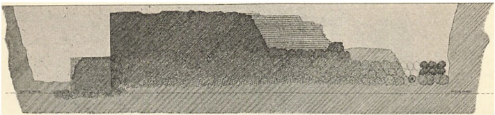
Snit gennem Blaataarn og Ringmuren, A—B.
