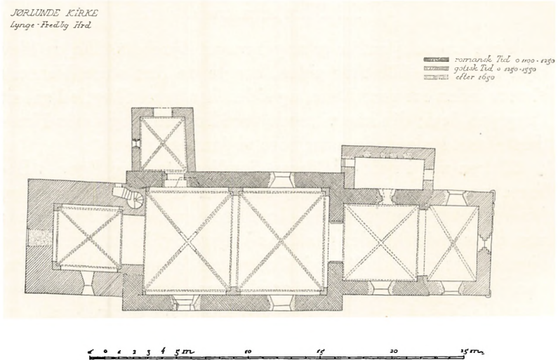
Jørlunde Kirke. Grundplan.
