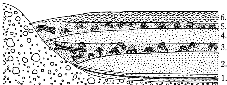
Skematisk Tværsnit af en nordsjællandsk Skovmose med Aflejringer fra samtlige Afsnit af Tidsrummet efter Istiden. — 1. Lerlag fra arktisk Tid med Gytjelag fra Allerødtid. — 2. Gytje og 3. Tørv fra boreal Tid. — 4. Gytje fra atlantisk Tid. — 5. Tørv fra subboreal Tid. — 6. Tørv fra subatlantisk Tid.
