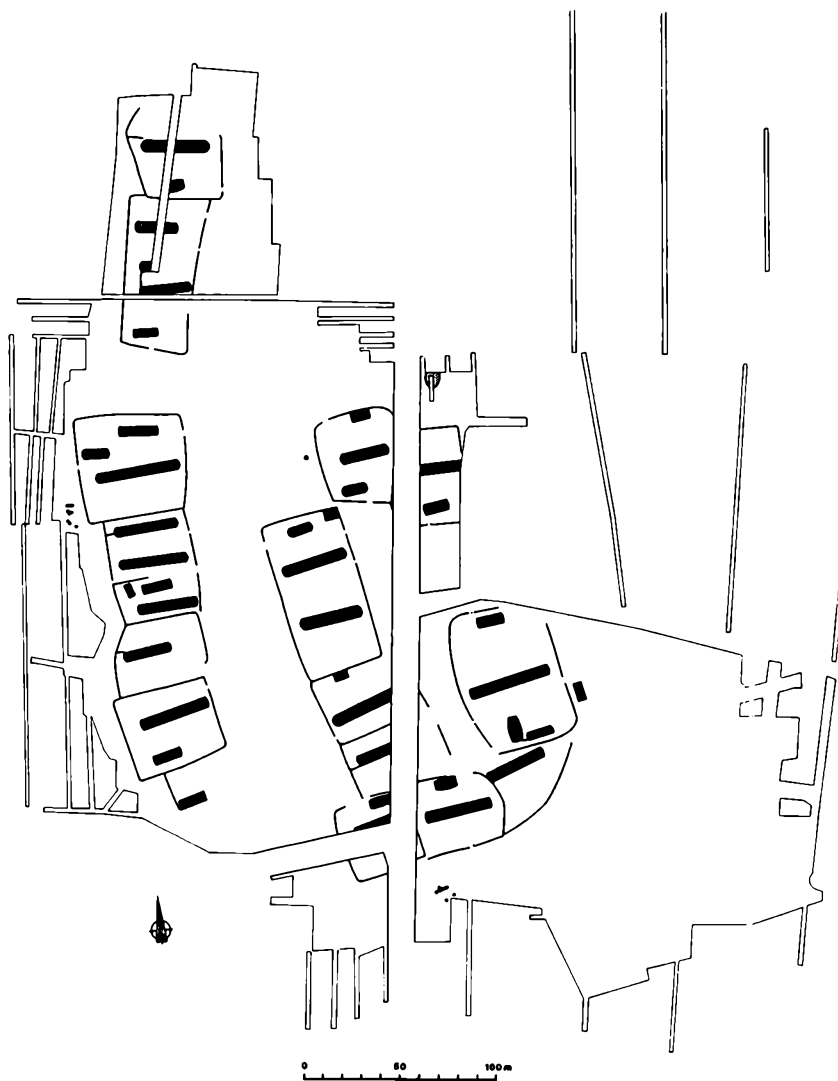
Fig. 6. Samlet plan af den samtidige landsby i 4. årh. e. Kr. f.
