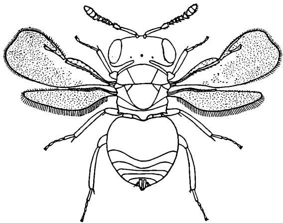
Simopterus Først. (orig.)
