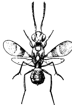
Anastatus Motsch. (after Bolivar y Pieltain)
