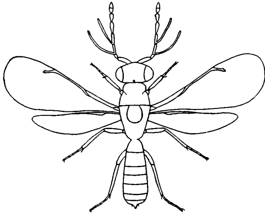
Dicladocerus Westw. (orig.)
