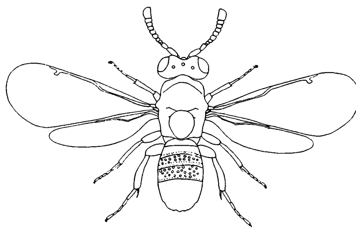
Ormyrus West. (orig.)
