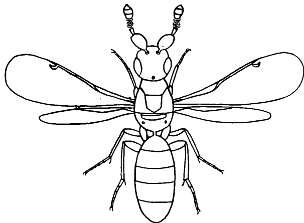
Pirene Hal. (orig.)
