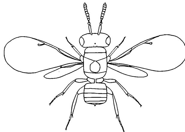
Habritys Thoms. (orig.)
