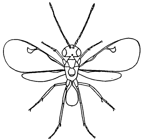
Miscogaster Walk (orig.)
