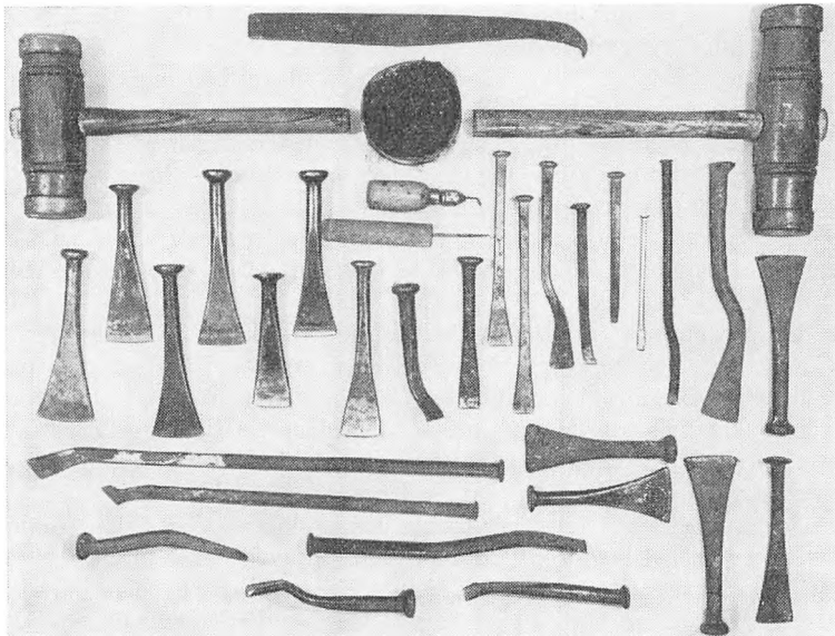
Til kalfatringen. Typesamling af jern og koller fra én bådebygger a .
