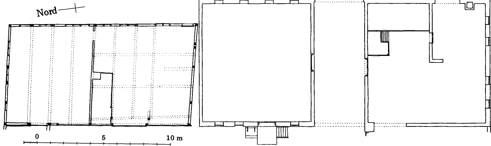
Baghuse Plan
