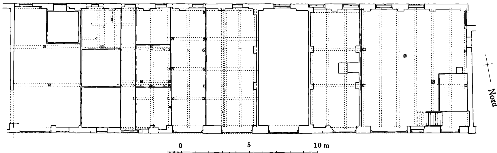
Magasinbygning Plan 1. etage
