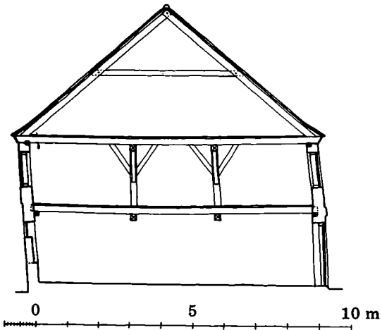
Magasinbygning Snit
