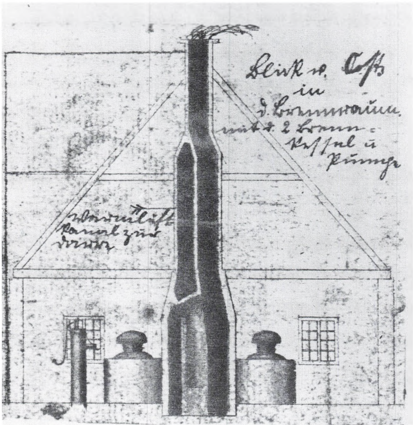
Tværsnit af brænderibygningen.
