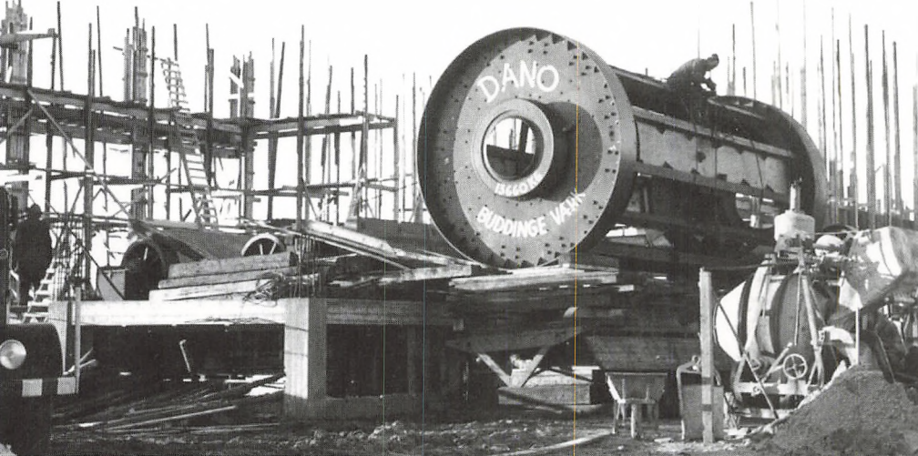
Århus Kommunes affaldsanlæg i Eskelunden under konstruktion. På den store komposterings-tromle ses DANO's logo.
