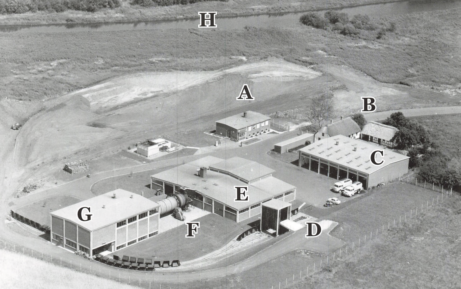
Eskelunden 1959 A=Administrationsbygningen, B= Gården Eskelund, C= Garageanlæg, D= Slaggesorteringsanlæg, E= Modtagelsesbygning, F= Silo til gæringsproces, G= Formalingen, H= Aarhus Å
