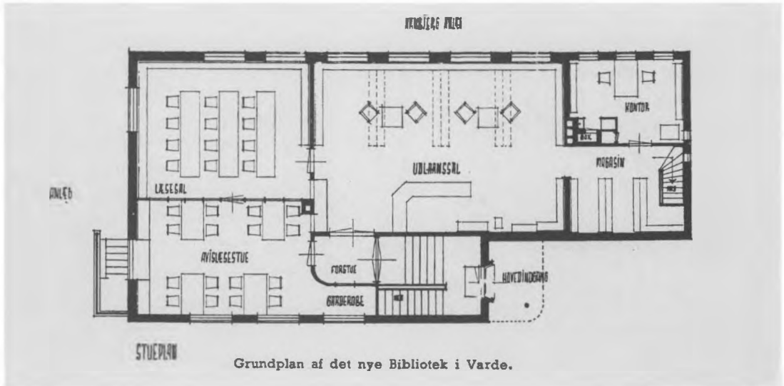
Grundplan af biblioteket på Lundvej. (Biblioteksårbog 1942)
