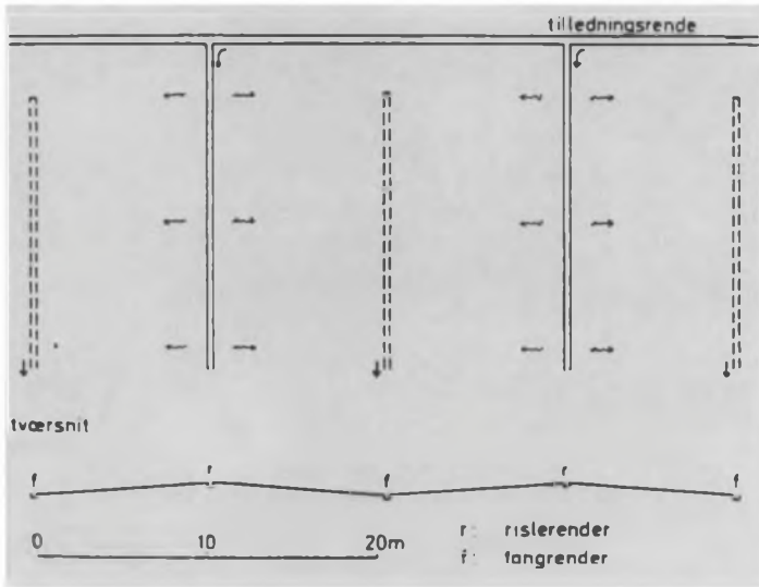
Tegning af del af tildannet ryglæg. Fra rislerenderne løber overskudsvand til de stiplede fangrender og derfra videre til andre anlæg eller til åen. Efter Søren Rasmussen: Store Skjernå kanal. 1985.
