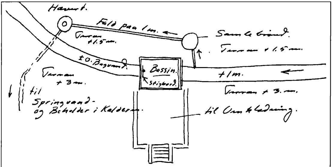
Badebassinet i bækken med vandværket, der gav mulighed for springvand i haven og vanding af kreaturerne i stalden. Tegning: Knud Høgsbro Østergaard.
