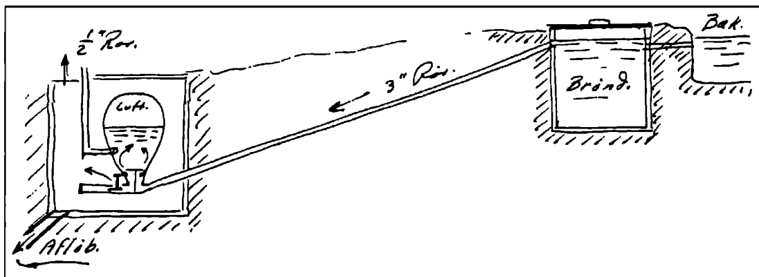
Tværsnit af hæverten i bækken. Tegning: Knud Høgsbro Østergaard
