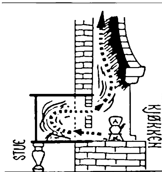
Bilæggerovnenes funktionsprincipper. Den forudsætter et åbent ildsted i et tilstødende rum – ofte køkkenet. Efter Hamran 1989 s 17.
