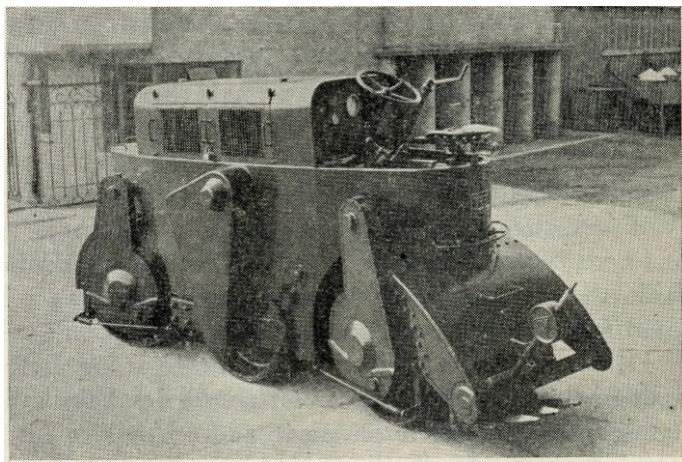
Et af "Pedershaab" Maskinfabrik's nyeste Fabrikata: Den verden spatenterede Vibrations-Vejtromle Type P M 7 A
