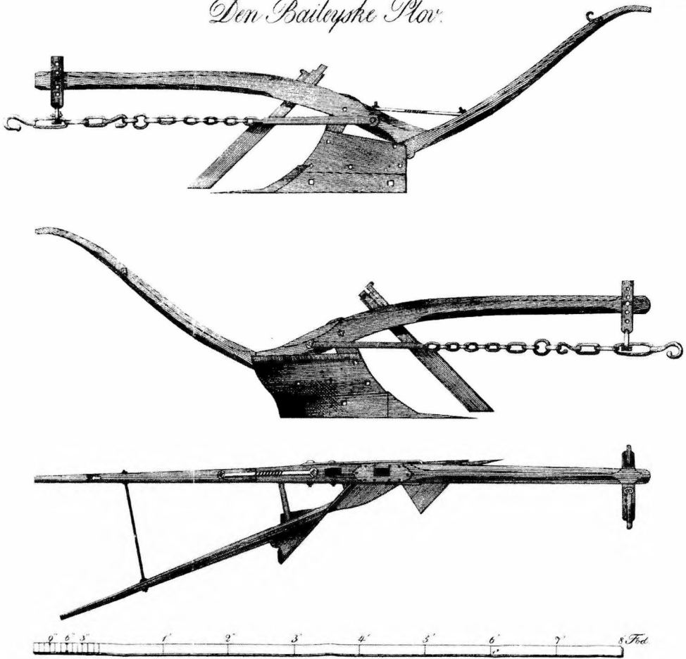
Den baileyske plov afbilledet i Nye Landoeconomiske Tiender, 1820. Fra: Dan Ch. Christensen: Det moderne Projekt, Teknik & Kultur i Danmark-Norge 1750-(1814)-1850, Viborg 1996.
