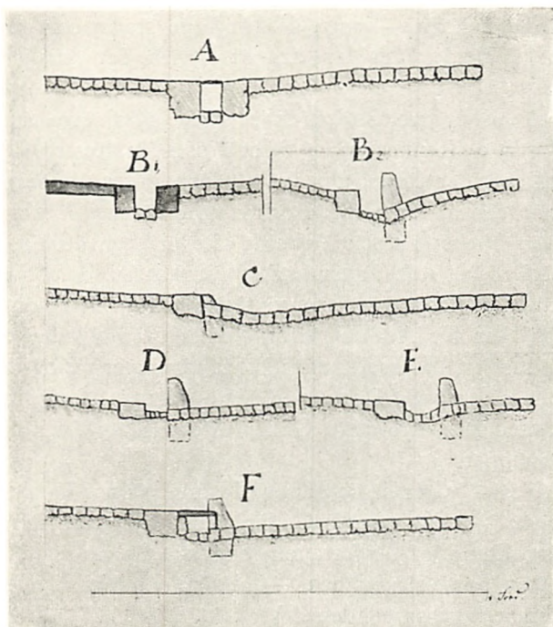
Fig. 4. Rendestentyper. Etter Tegning 1776.
