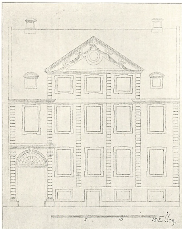
Fig. 6. Typetegning til mere anseligt Borgerhus. (Efter Krieger 1729).
