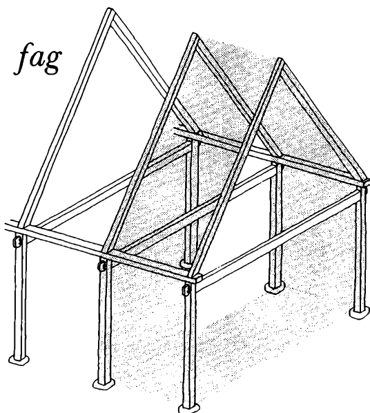
Tegning af »fag« fra Grith Lerche: Bøndergårde i Danmark 1789–90 . 1987. Bygningens størrelse blev angivet ved deres antal fag i længderetningen.
