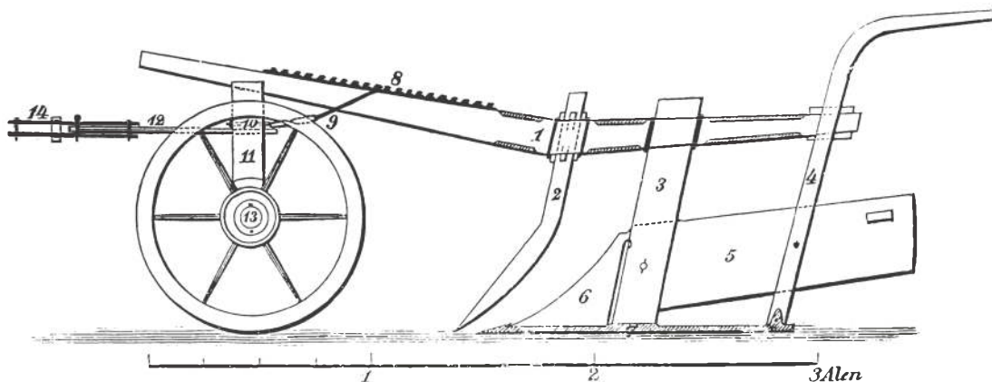
Gammel sønderjydsk hjulplow. 1: bom eller ås; 2: langjern; 3: sulen; 4: håndved; 5: muldfjæl; 6: muldplade; 7: skære; 8: bom- eller åstammen; 9: skaftet; 10: skruestammen; 11: skruen; 12: tungen; 13: urlen; 14: skankloven.
