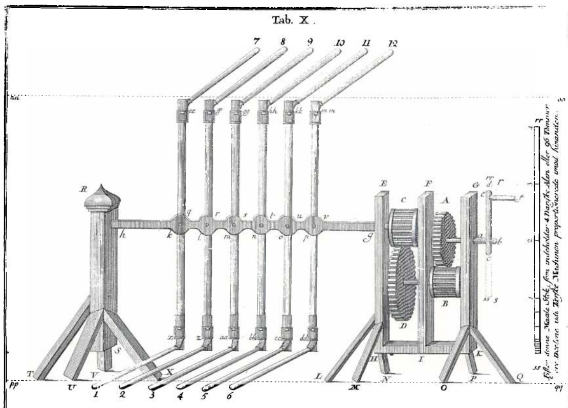
Tegning af en maskine, »som tjener til at tærsk kornet, i det mindste på vore store avlsgårde, således at 6 à 8 karles arbejde derved spares, og såvel strå som korn dog behandles lige vel«.
