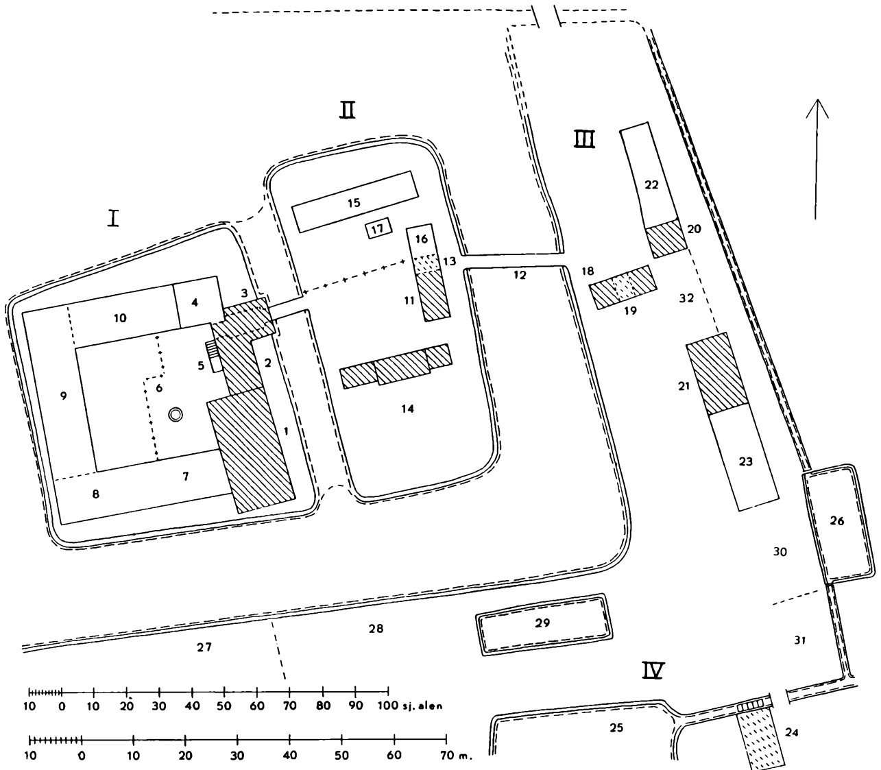
16. Clausholm, som Mogens Gøyes arvinger modtog det 1546. Planen viser skitse-mæssigt, hvorledes Clausholm må tænkes at have set ud 1546, og det er angivet, hvad der ved første deling tilfaldt dels Albrecht (ikke skraveret) og dels Eline, der var repræsenteret af sin mand Mourids Oisen Krognos (skraveret). Skiftebrevet (jfr. note 67) meddele herom:
