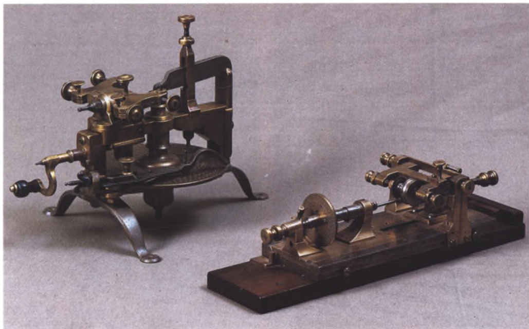
Fig. 22: De to inddelingsmaskiner, som Rønne Urmagerinteressentskab i 1894 forærede til Bornholms Museum, den venstre til skæring af tandhjul, den højre til skæring af drev.
