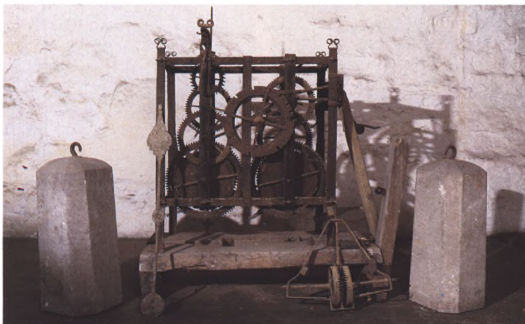
Fig. 21: Tårnurværk, lavet i Poulsker i 1821 af tidligere urmager i Neksø Jens Larsen til Neksø Kirke. Nu ude af brug og hensat på kirkeloftet. Ved siderne er anbragt de tilhørende lodder af sten.
