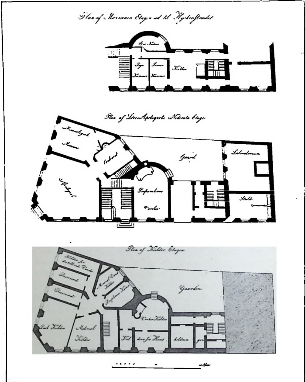
Grundplener til den for Løve-Apoteket i København 1796—98 opførte Ejendom. Efter Tegninger af C. F. Harsdorff (49)
