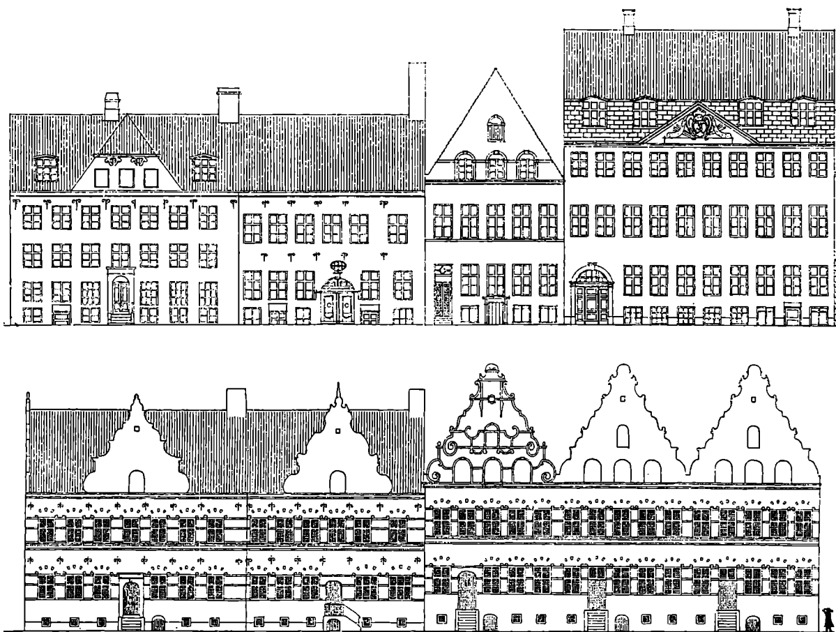
Strandgade Nr. 32—36. Foroven Husenes Tilstand o. 1940, forneden Rekonstruktion af deres oprindelige Udseende o. 1640. Opmaalinger af H. H. Engquist.
