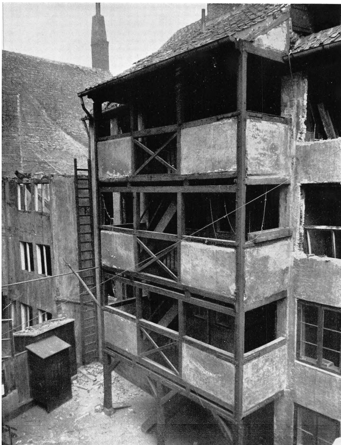
Udvendigt Trappe-Anlæg i tre Stokværk fra 1700'erne i Vognmagergade-Kvarteret. Nu nedrevet.
