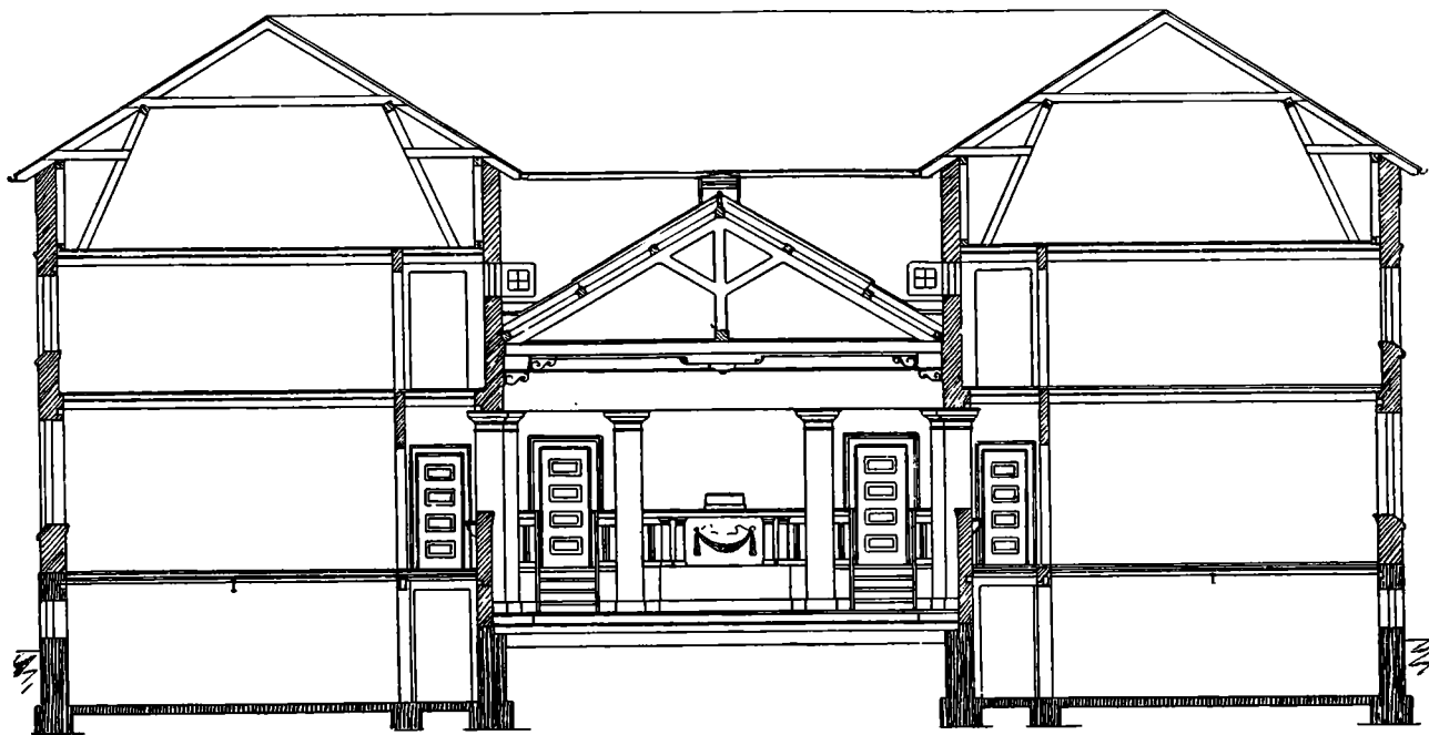
Snit gennem Huset, der viser Etagerne og Foredragssalen i den overdækkede Gaard.
