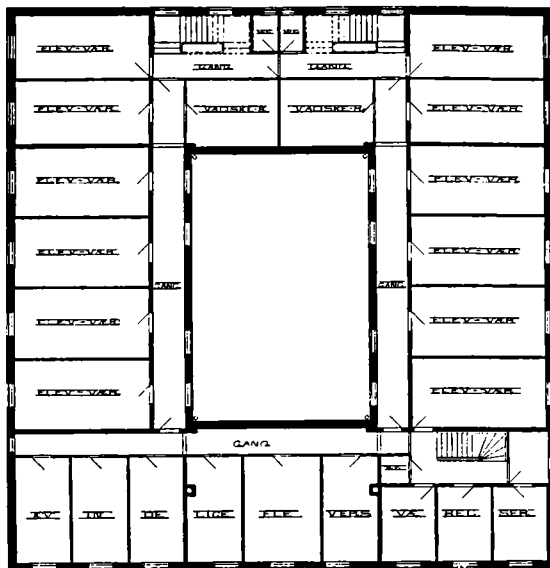
Grundplan af 1. Sal.
