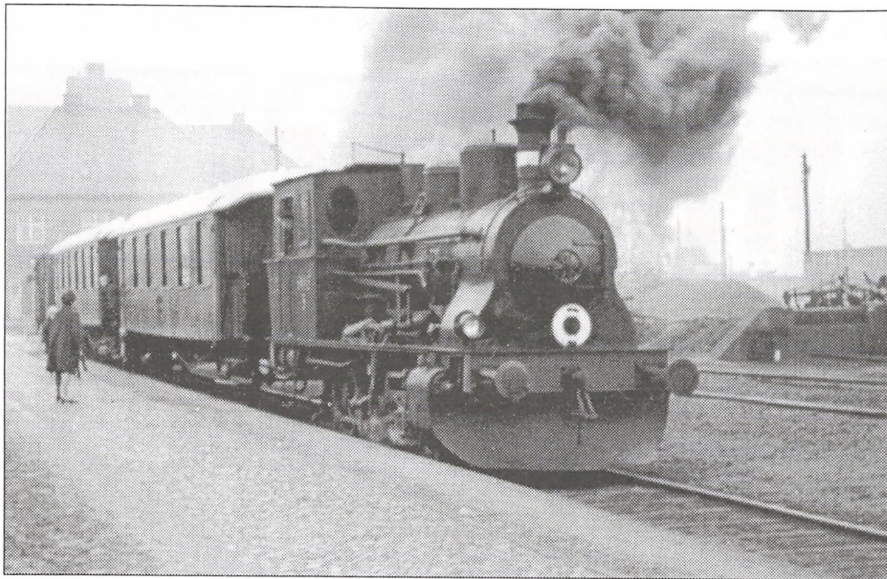
Stubbekøbing-Nykøbing-Nysted-Banen åbnede 1911
