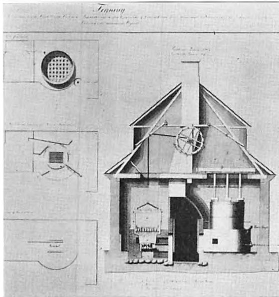
Fig. 23. »Tegning over de 1824 indrettede tvende Vand-Damp-Vaskningsapparater udført efter Opgivelse af Kommissionen, som allernådigst har været befaleet til Forslag med Vand-Damp-Vaskning på Almindeligt Hospital«.
