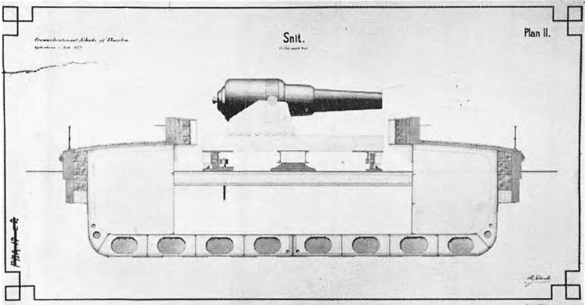
Tværsnit af senere marineminister Jönckes udkast til et flydende fort efter engelsk forbillede. Fortet var forsynet med 3 kanoner.
