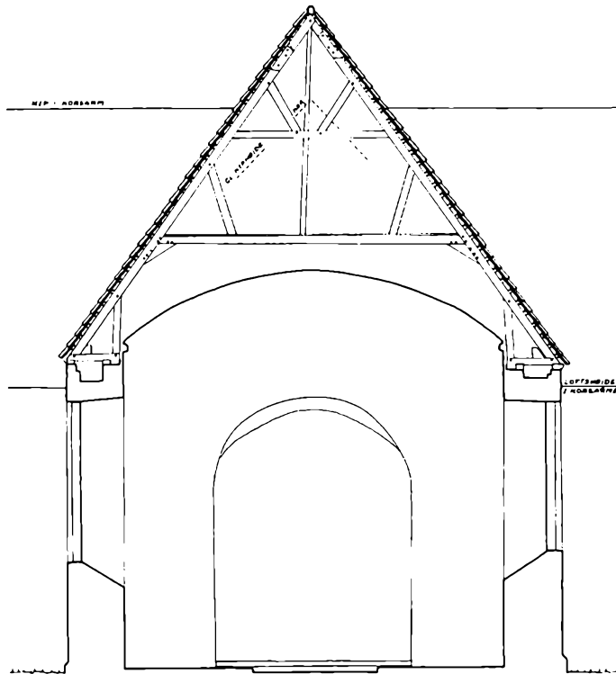
Fig. 8. Tværnsnit gennem skib, set mod øst, 1:150. Målt af SGP 1977, tegnet af MN 1984. – Querschnitt durch das Schiff.
