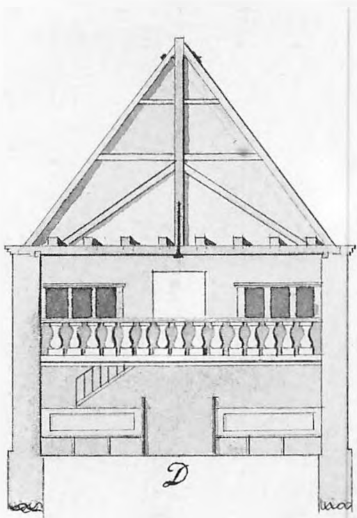
Fig. 37. Korsarmspulpitur o. 1810 (s. 916) med samtidige flukkede stole (nr. 7-10, s. 916). Udsnit af Mikkel Stobberups indretningsforslag 1808 (fig. 12) i LA Vib. — Kreuzarm-Empore um 1810 mit fgeschlossenen Stühlen aus der gleichen Zeit (Nr. 7-10). Ausschnitt aus Mikkel Stobberups Einrichtungsvorschlag 1808.
