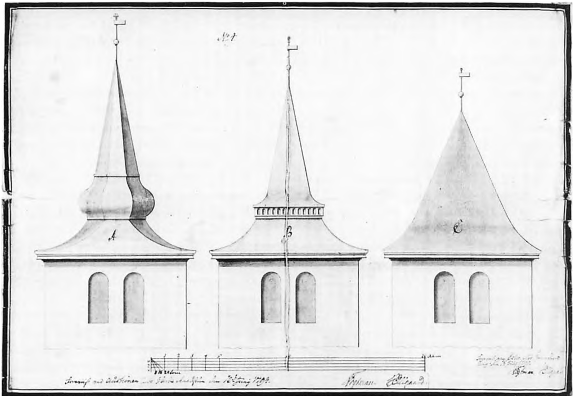
Fig. 6. Forslag til spir over tårnet, tegnet af Mikkel Stobberup 1794. Det midterste forslag, B, blev udført (s. 948). Mål i danske alen. Farvelagt tegning i Landsarkivet for Nørrejylland. — Vorschläge zu einer Turmspitze, entworfen von Mikkel Stobberup 1794. Der mittlere Vorschlag, B, wurde ausgeführt. Maße in dänischen Ellen.
