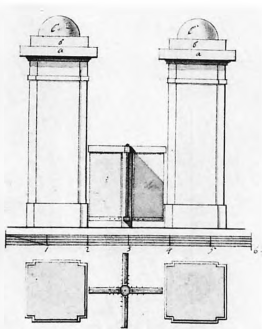
Fig. 3. Forslag til kirkegårdsindgang, tegnet af Mikkel Stobberup 1796 (s. 945). Mål i danske alen. Landsarkivet for Nørrejylland. — Vorschlag zum Friedhofseingang, entworfen von Mikkel Stobberup 1796.
