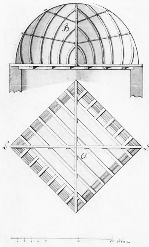
Fig. 15. Mikkel Stobberups forslag 1808 til tagværket i tårnets kuppel (s. 886). Farvelagt tegning i Landsarkivet for Nørrejylland. — Mikkel Stobberups Vorschlag von 1808 zur Überdachung der Kuppel des Turms.
