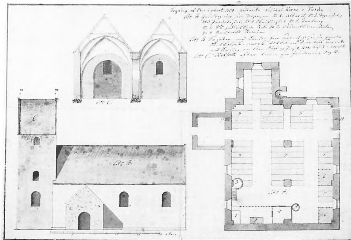
Fig. 4. Kirken før nedrivningen 1809, vist med det gamle tårn, som 1794 afløstes af spir. Grundplan (vest opad), tværnsnit set mod vest og opstalt af sydfacaden. Tallene 1-8 på grundplanen angiver: 1. Alter. 2. Degnestol. 3. Prædikestol. 4. Skriftestol. 5. Døbefont. 6. Lukkede stole. 7. Fruentimmerstole. 8. Mandfolkestole. Mål i danske alen. Tegning i Varde byhistoriske arkiv. — Die Kirche vor dem Abbruch im Jahr 1809, dargestellt mit dem alten Turm, der 1794 von einer Turmspitze abgelöst wurde. Grundriß (Westen oben), Querschnitt gegen Westen gesehen und Aufriß der Südfassade. Die Zahlen 1-8 auf dem Grundriß geben an: 1. Altar. 2. Küsterstuhl. 3. Kanzel. 4. Beichtstuhl. 5. Taufe. 6. Geschlossene Gestühle. 7. Frauenzimmerstühle. 8. Männerstühle. Maße in dänischen Ellen.
