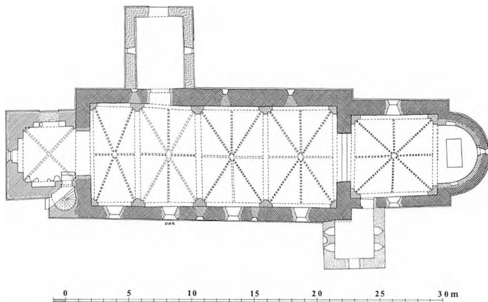
Fig. 4-5. Grundplan 1:300 og tværsnit 1:150 gennem skib. Målt af Henrik Gram og Søren Gottfred Petersen 1978, tegnet af MN 1985. — Grundriß 1:300 und Querschnitt 1:150 durch das Schiff.
