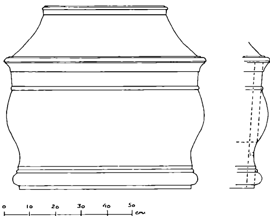
Fig. 4. Peter Rodsteens († 1714) kiste i Århus Domkirke. Snedkret af Johan Schumacher og udsmykket af Nicolai Schrøder. Fodende målt og tegnet af Niels J. Poulsen 1975
