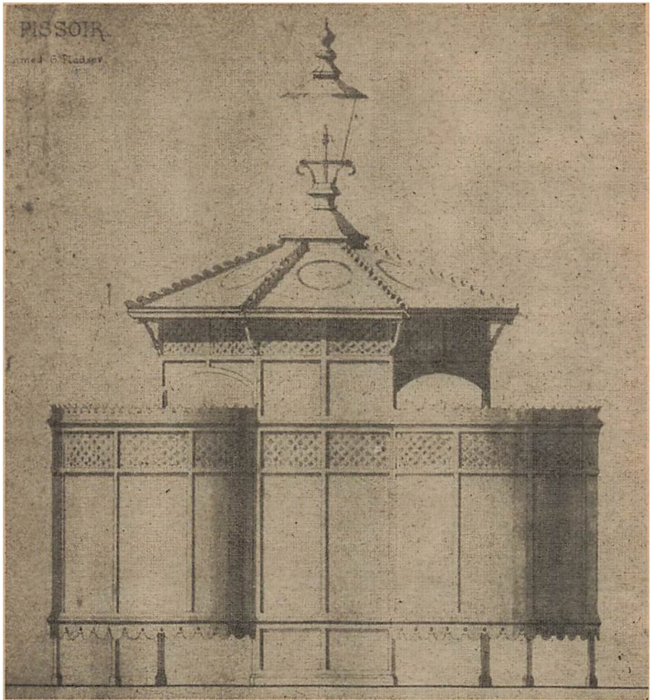
Udformningen af et pissoir var en alvorlig opgave. Dette etablissement er tegnet af teaterarkitekten V. Dahlerup, dateret november 1891 (Vejkontoret, Stadsingeniørens Direktorat). Tegningen er betegnet »Pissoir med 6 Pladser«; der blev også skitseret typer beregnet på færre personer.
