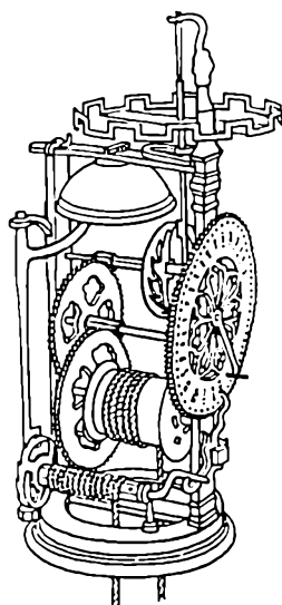
Fig. 21 Vækkeur fra et kloster
