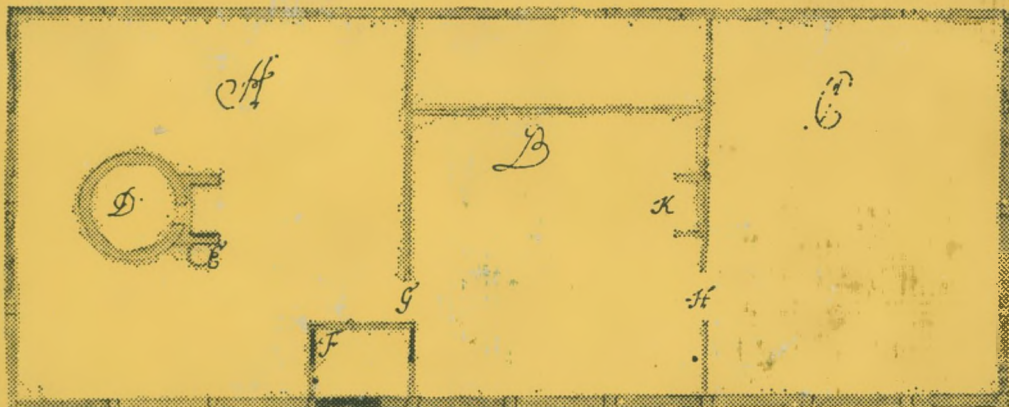
Gründ Tegning paa Vaaringshuus bestaaende af 10 Væg.
