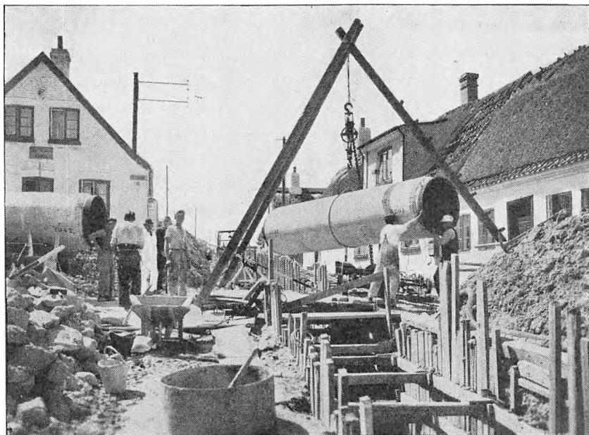
Staalbeton-Rør til den københavnske Vandledning nedlægges i Brøndgade.
