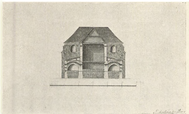
Fig. 3. Tværsnit af Nikolai kirke, set mod øst.
