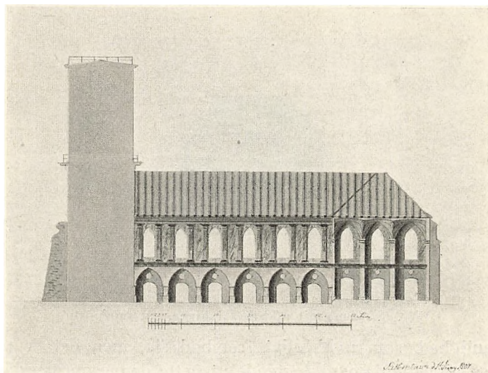
Fig 2. Længdesnit af Nikolai kirke.
