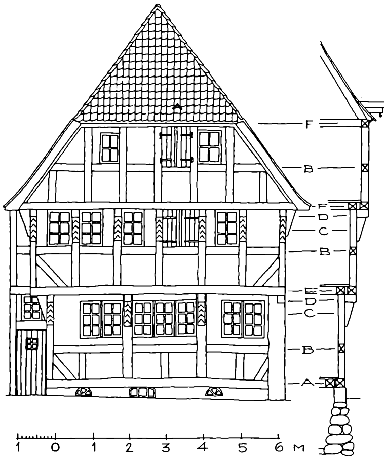
Fig. 7. Facade mod gården til ejendommen matr. nr. 448A, Storegade. Nedtagen 1917. A=Fodrem. B=Fylldholt. C=Knægt. E=Overgangsod. F=Tagrem.
