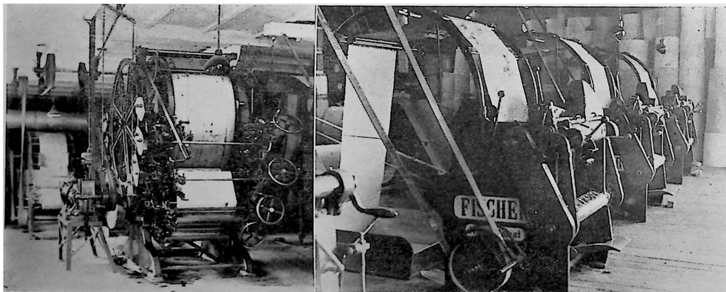
Elektrisk drevet 8-farvet Trykautomat.
