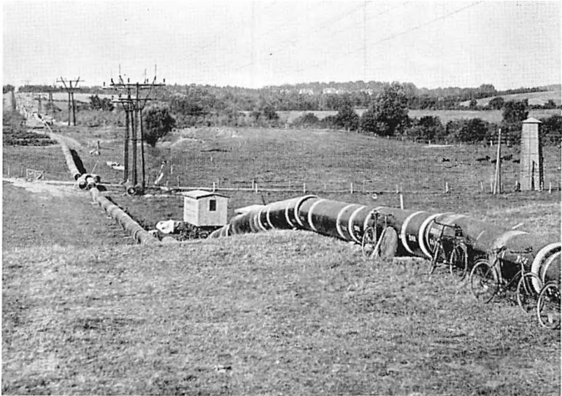
Lægning af Ledningen fra Sjælsø Vandværk.
