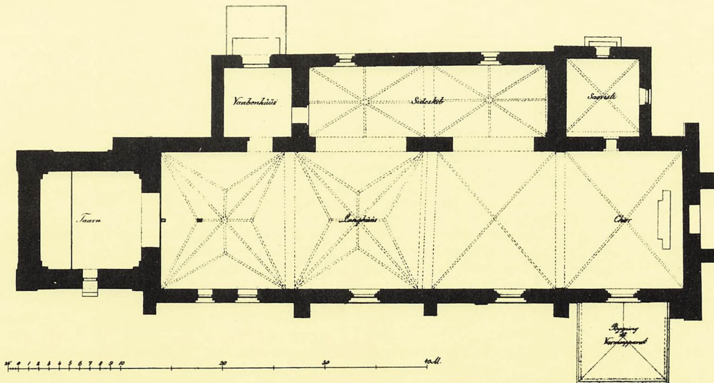
Grundplan af den gamle kirke.
