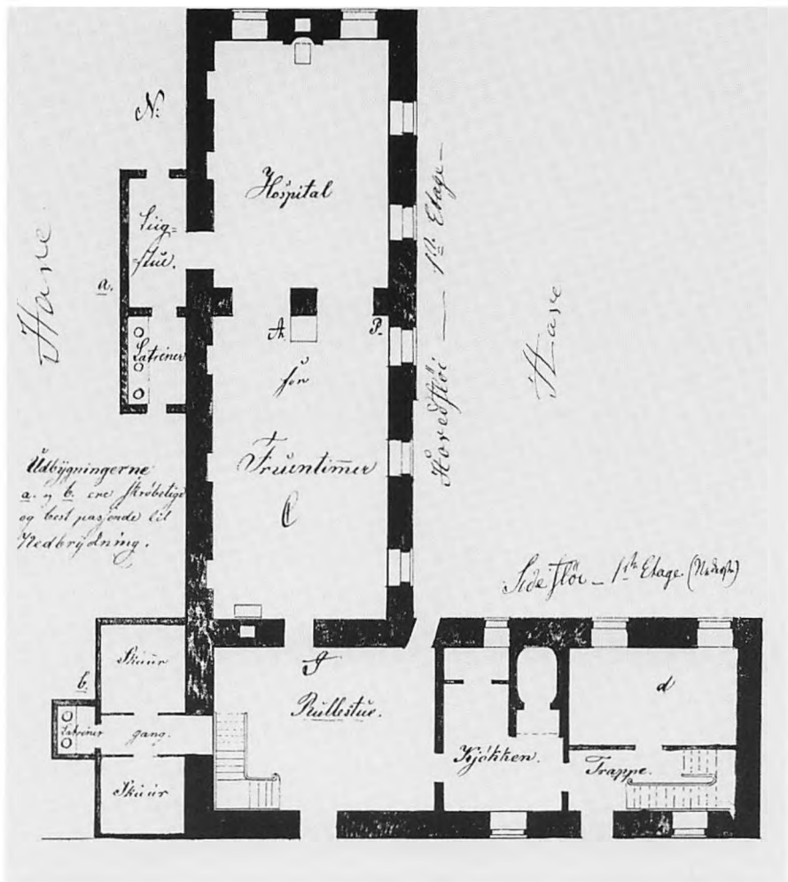
Da man første gang, i 1819, spekulerede på en ombygning af Hospitalet, lavede murermester Lars Grønbæk (1773-1854) en nøjagtig grundtegning; her er kun stueetagen vist. I hovedstøjen (C) er der hospital for fruentimmer, A står for alter og P for prædikestol. På nordsiden er der tilbygget ligstue og latriner. I sydstøjen genkender man den store bageovn. Ved nordgavlen er tilbygget to skure med gang og latriner; det drejer sig om dårekisterne. Alle tilbygningerne betegnes som skrøbelige og bedst passende til nedbrydning. Justitsministeriets arkiv. Rigsarkivet.
