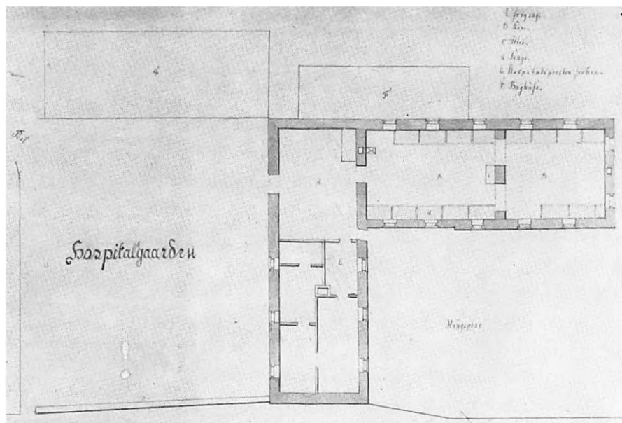
Grundplanen af Hospitalet er tegnet af Chr. Gullep så sent som i 1885, men viser i hovedtrækkene, hvordan Hospitalet så ud i 1600-årene; det gælder dog ikke sydfløjen, hvor hospitalspræstens lejlighed er markeret. A. Forgang. B. Stuer. c. Alter. d. Senge. F. Baghuse. Sammenhold også med tegningen indvendig på bagflappen. Viborg Stiftsmuseum.
