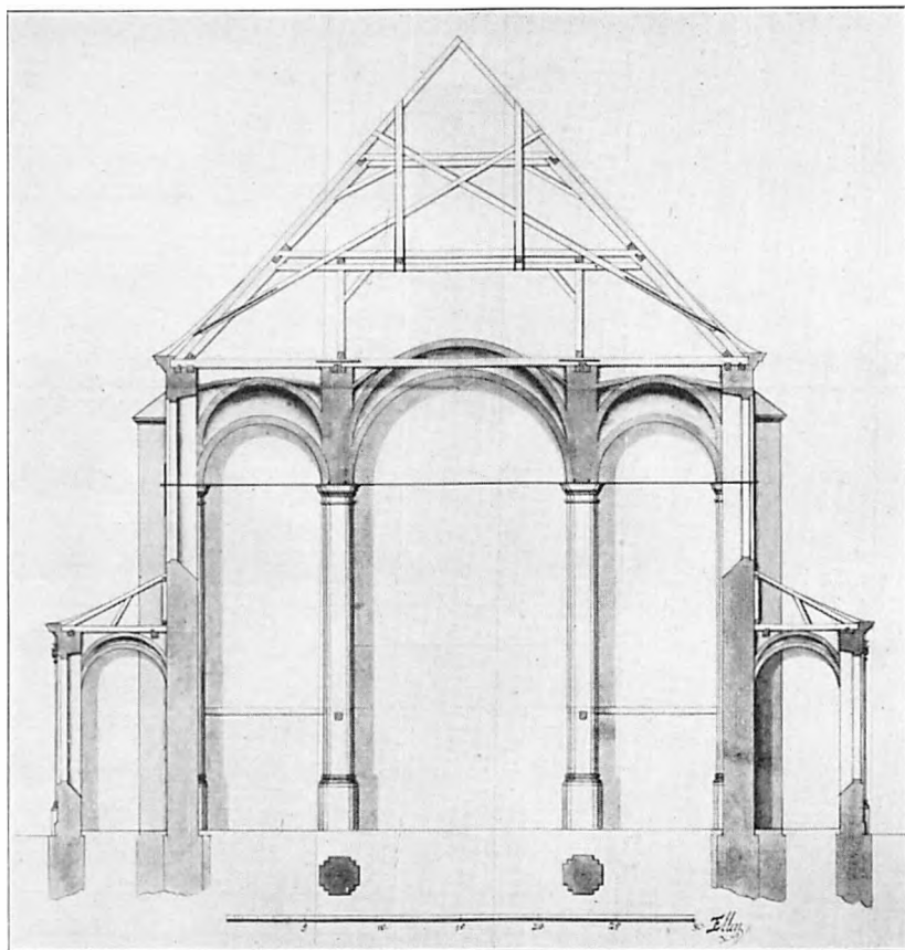
Afb. 26. Tværsnit af Kirken. J. G. Kreyslg del. Bogsarkivet.
