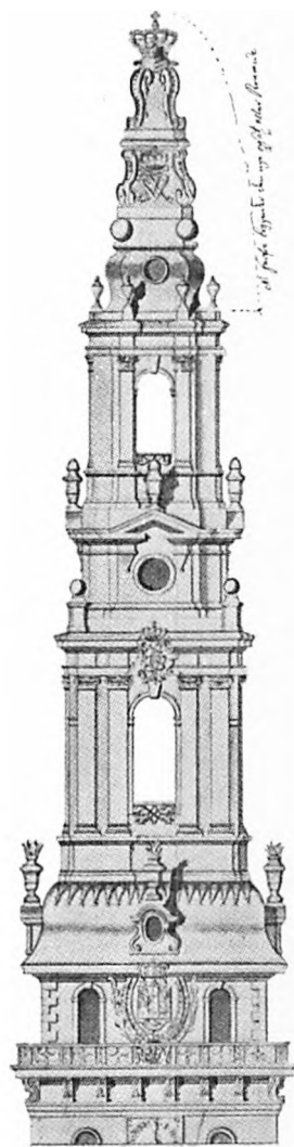
Afb. 28. L. Thuras Forslag til Forkortning af Spiret. L. Thurn del.
