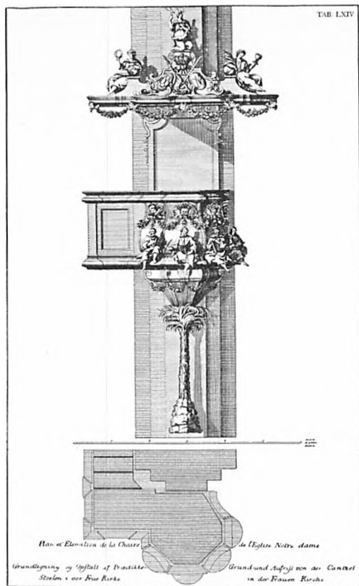
Afb. 32. Prædikestolen. Efter L. Thurn: Den danske Vitruvius.
