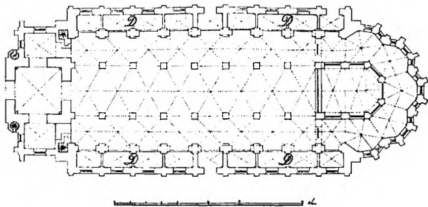
Afb. 5, 6. J. F. Ramus' Projekt til Kirkens Genopfoelse. 1731. Rigsarkivet.
