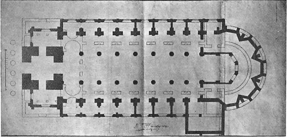
Afb. 36. Plan af den 1807 nedbrændte Kirke, med indtegnet Projekt til den nye. Universitetsbibliotheket. C. F. Hansen del.
