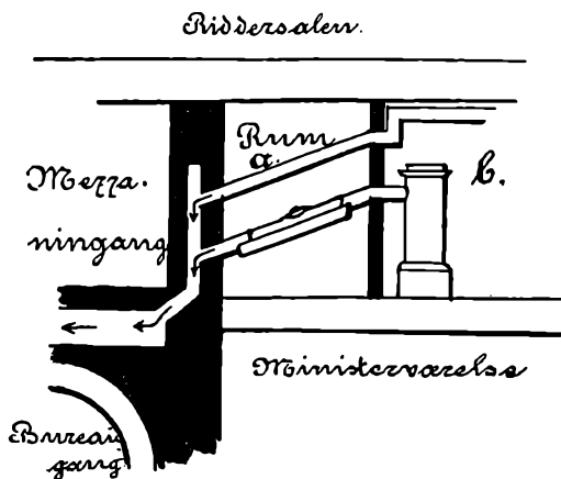
Snit gennem Værelset, hvor Ilden opstod.
